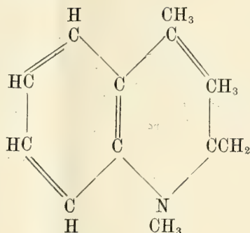
Trimetildiidrochinolina.
